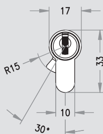
Modulbauweise
